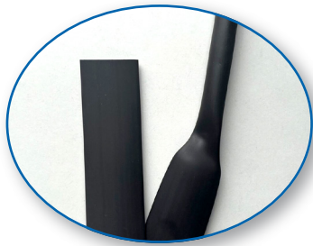
TRPF-DR Tubos termorretráctiles Diesel Resistant Pared fina / Sin adhesivo Contracción 2:1 Temperatura de trabajo -75° C a 150° C
