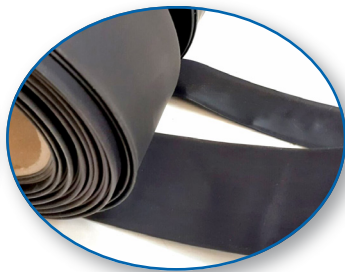
TRPF150°C Tubos termorretráctiles Poliiolefina Pared fina / Sin adhesivo Contracción 2:1 Temperatura de trabajo -55° C a 150° C
