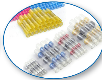
CTRAD Y CTRES Conectores termorretráctiles Con adhesivo Temperatura de trabajo -45° C a 125° C Conectores termorretráctiles Con anillos y estaño Temperatura de trabajo -55° C a 125° C
